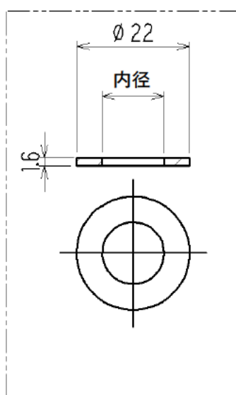
垫片
