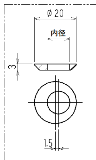
夹紧垫片
